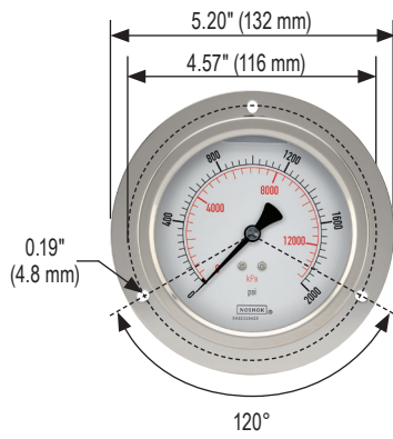
40-911 Front Flange
