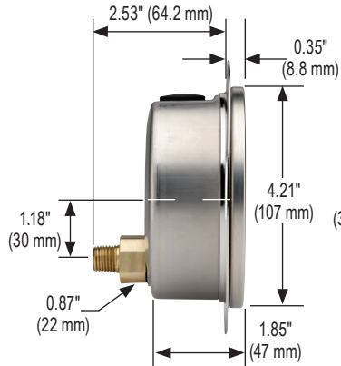
40-911 Front Flange
